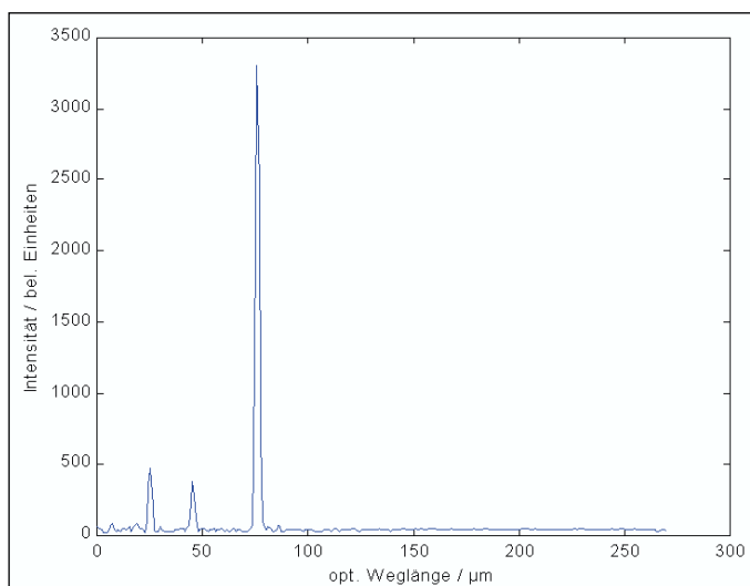
Abb. 3: Fouriertransformiertes Spektrum bei Messung eines Zweischichtensystems.
